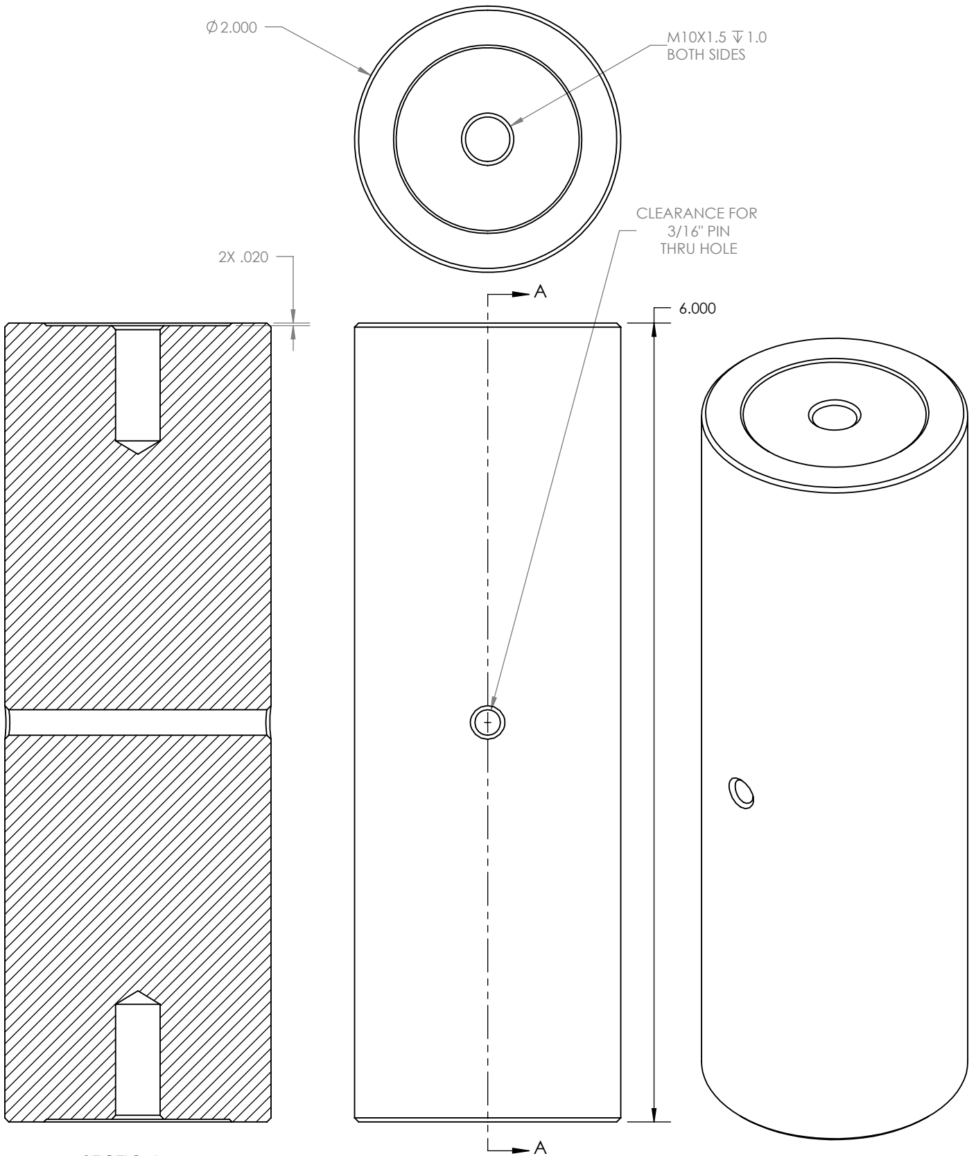
SECTION A-A
